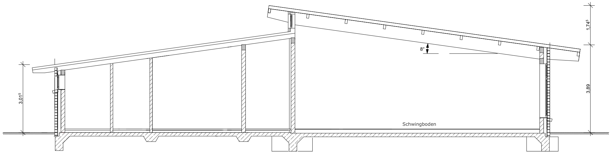
Schnitt A-A
